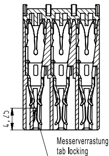
Verrastung für Flachsteckmesser locking feature for tabs
