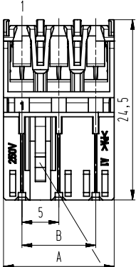
Verrastung für Flachsteckmesser locking feature for tabs
