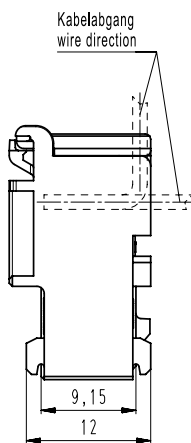
Innenverrastung inside locking
