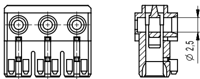
Darstellung ohne Kontakte Designation without contacts
