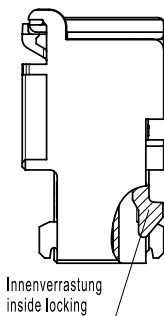
Messerverrastung tab locking
