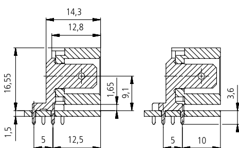
Platinenrand PCB edge
